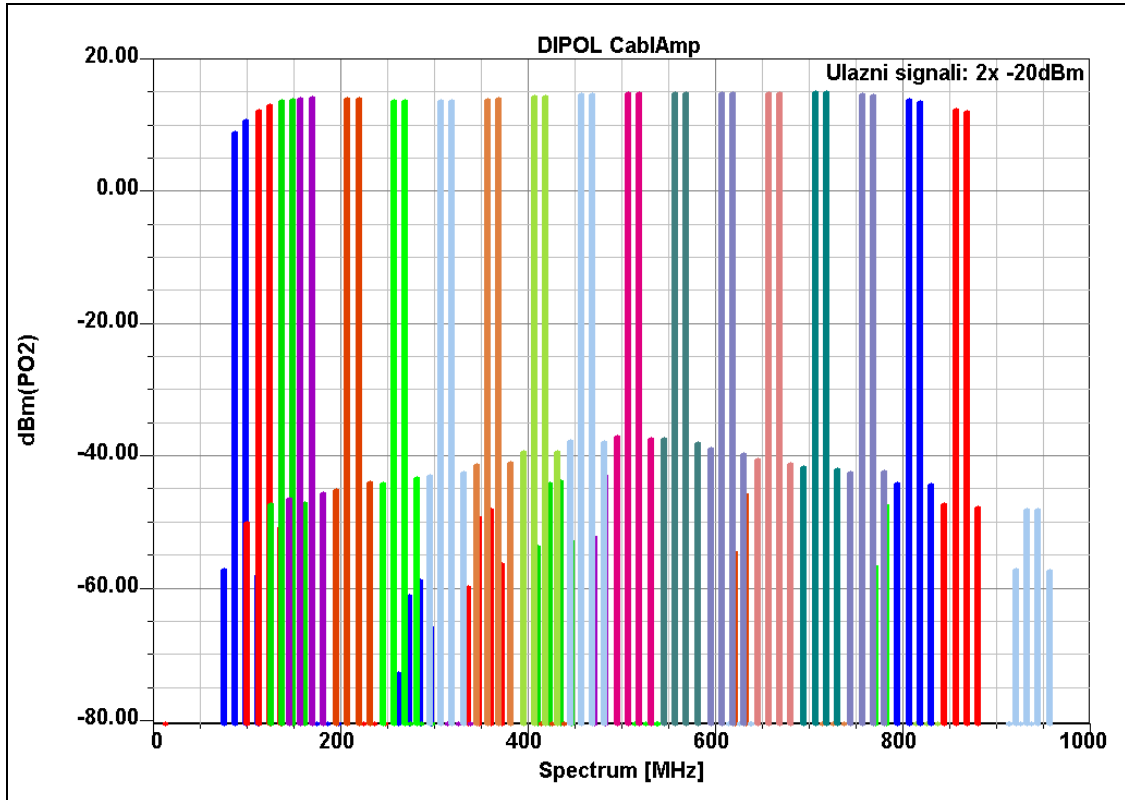
Tipican spektar dvotonskog signala na razlicitim parovima frekvencija
