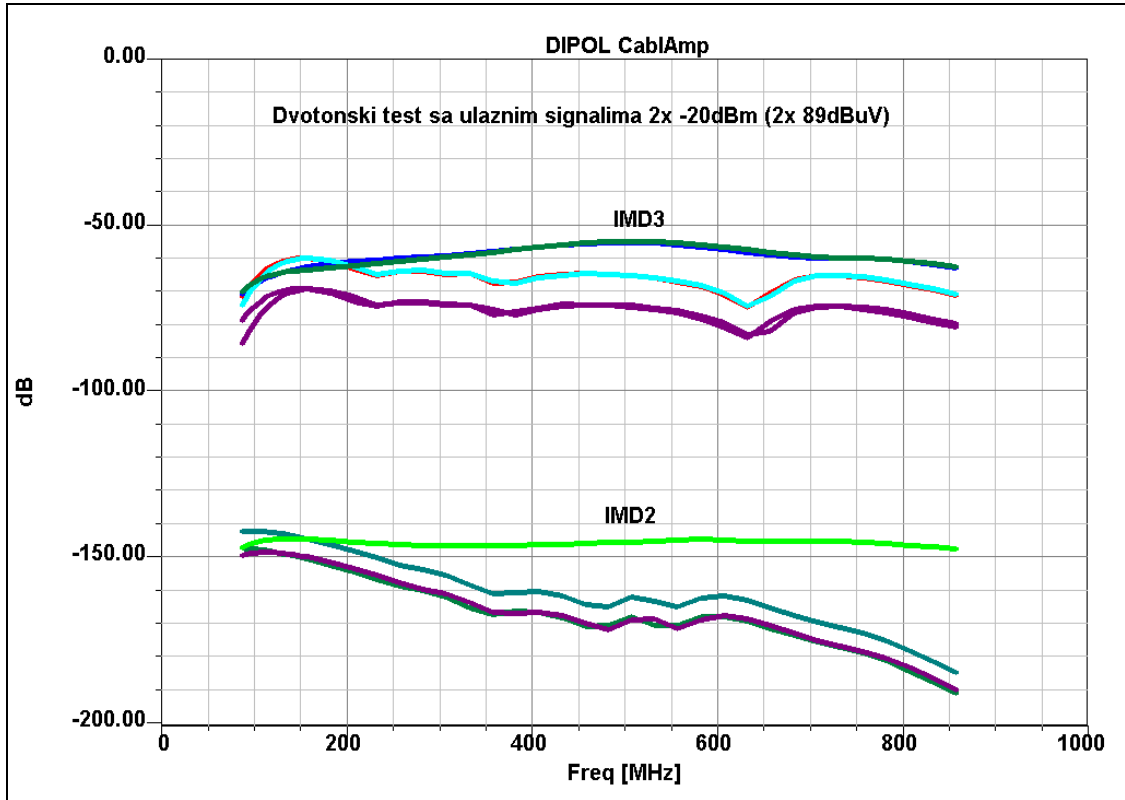
Tipicna kriva IMD produkata za pojačavac bez ekvilizacije
