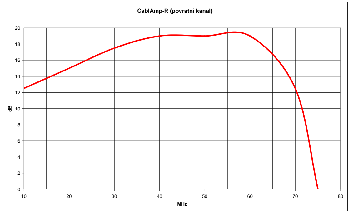
Tipicna kriva pojačanja povratnog kanala
