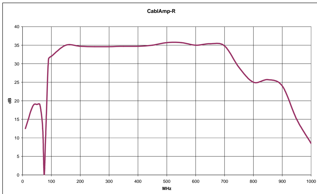
Tipicna kriva pojačanja bez ekvilizacije
