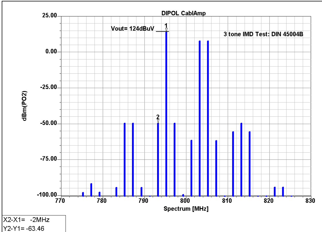
Tipican spektr trotonskog signala prema DIN 45004B testu
