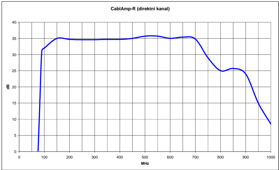
Tipicna kriva pojačanja direktnog kanala
