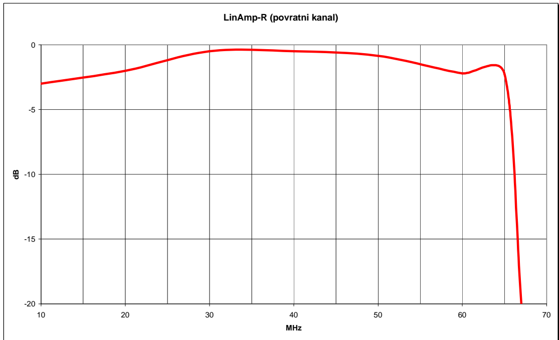
Tipicna kriva slabljenja pasivnog povratnog kanala
