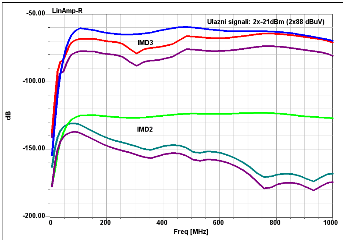
Tipična kriva IMD produkata za pojačavac bez ekvilizacije
