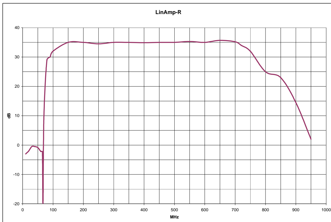
Tipicna kriva pojačanja bez ekvilizacije
