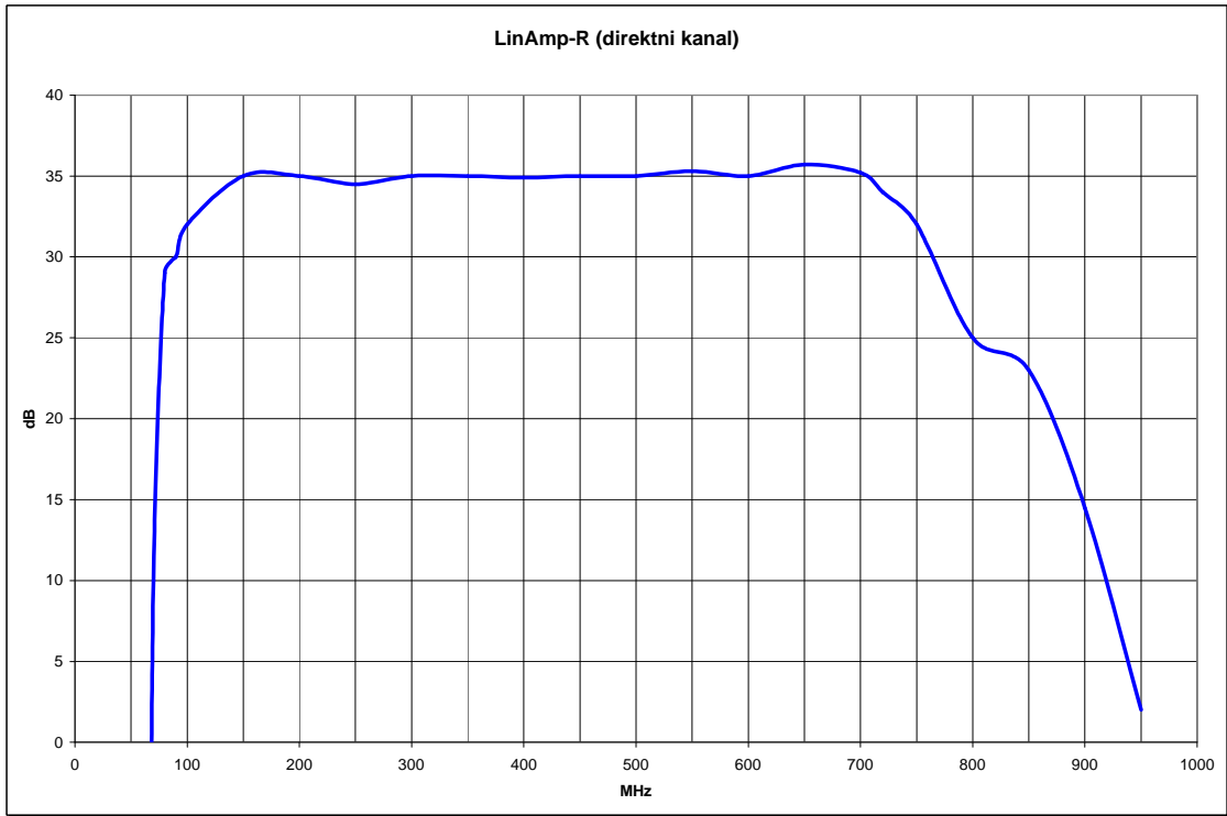
Tipicna kriva pojačanja direktnog kanala
