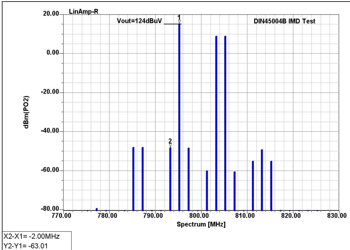
Tipican spektr trotonskog signala prema DIN 45004B testu
