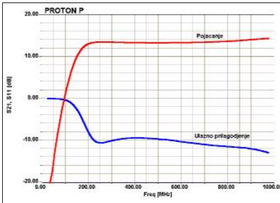
Tipična kriva pojačanja i ulaznog prilagođenja
