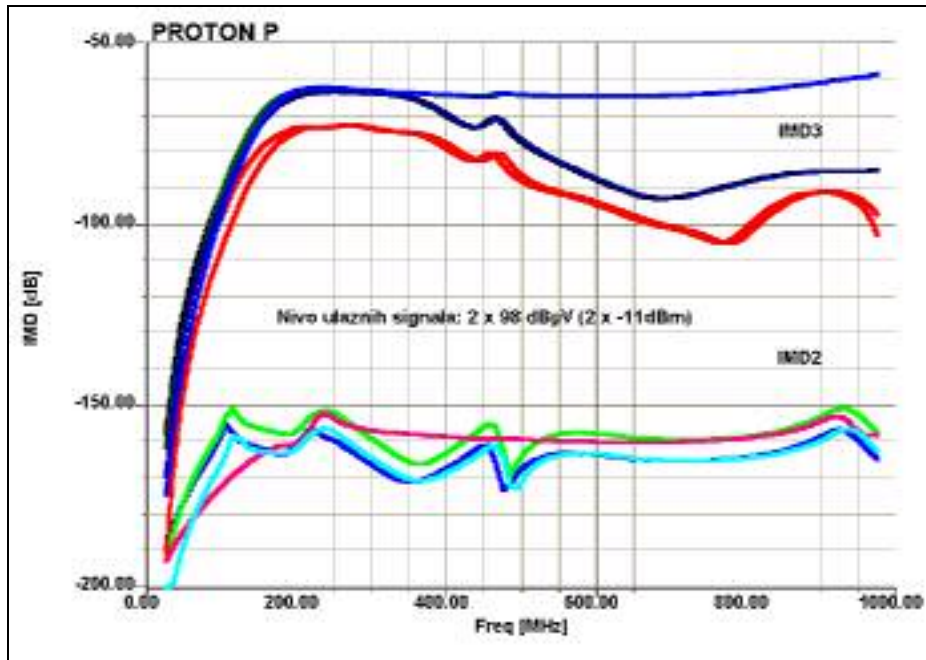
Tipična kriva IMD produkata za pojačavač pri dvotonskom testu
