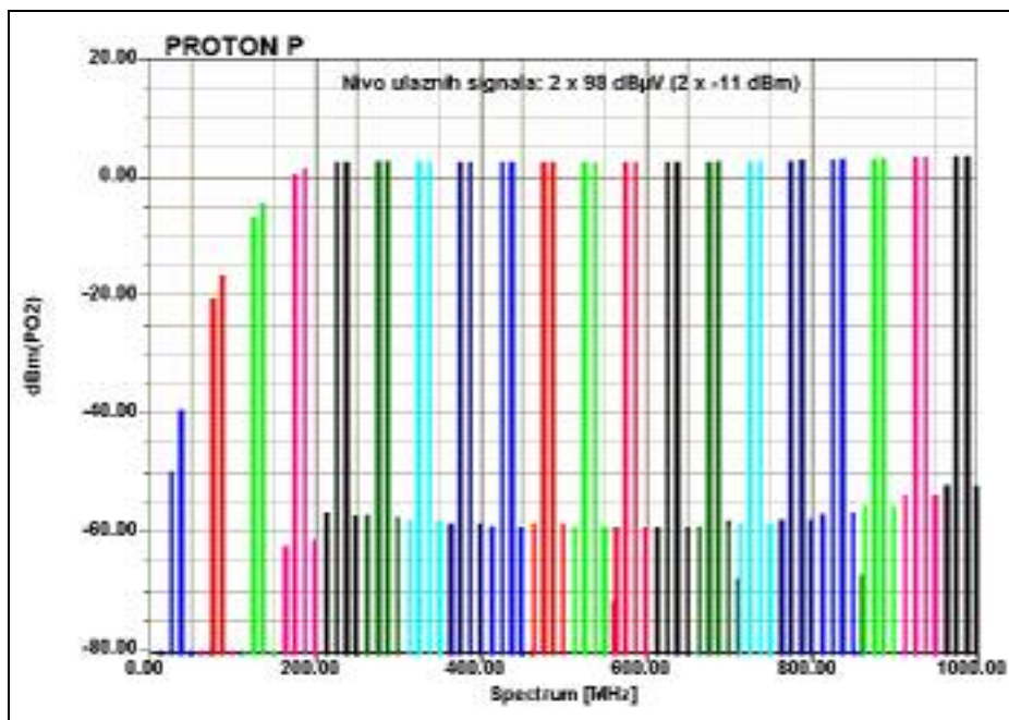
Tipičan spektar dvotonskog signala na različitim parovima frekvencija
